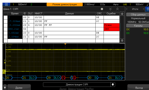
Рисунок 16 Запуск по сигналу и декодирование протокола CXPI
