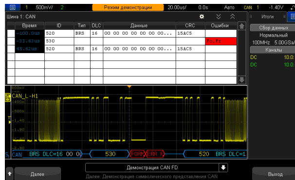
Рисунок 15 Запуск по сигналу и декодирование протокола CAN FD
