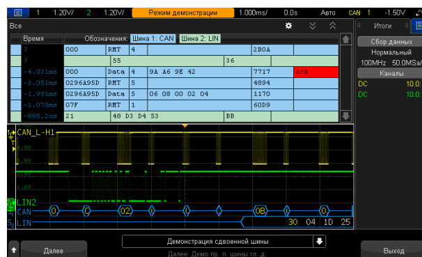
Рисунок 17 Запуск по сигналу и декодирование протокола двуденной ШИНЫ
